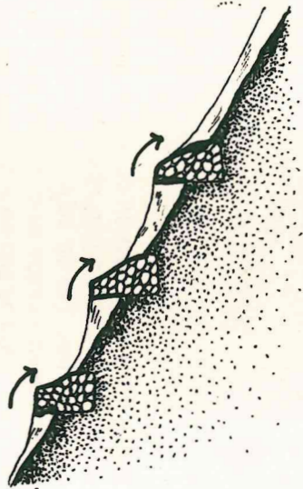
Sección transversal mostrando los saltos hidráulicos mediante muros bajos.
