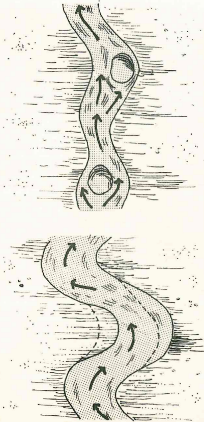
Corrección de curvaturas: Esquema de corrección del cauce sinuoso de una torrentera. Derecha, limpieza del cauce en una torrentera.
