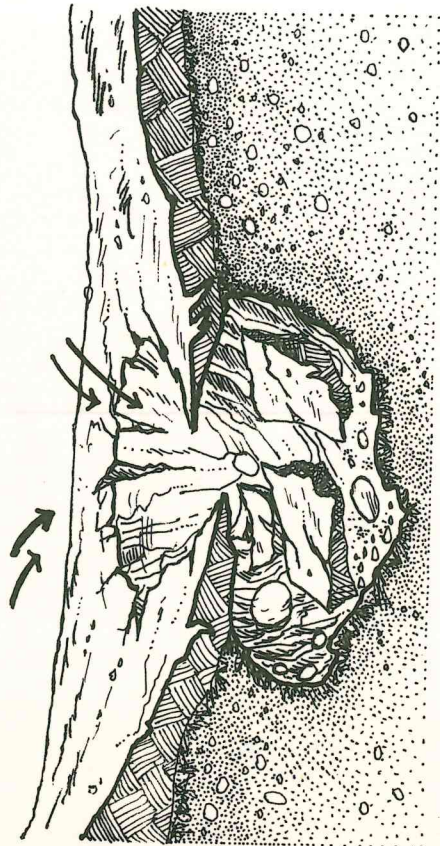
Ilustración de hundimiento y colapso de una caverna por disolución de calizas.
